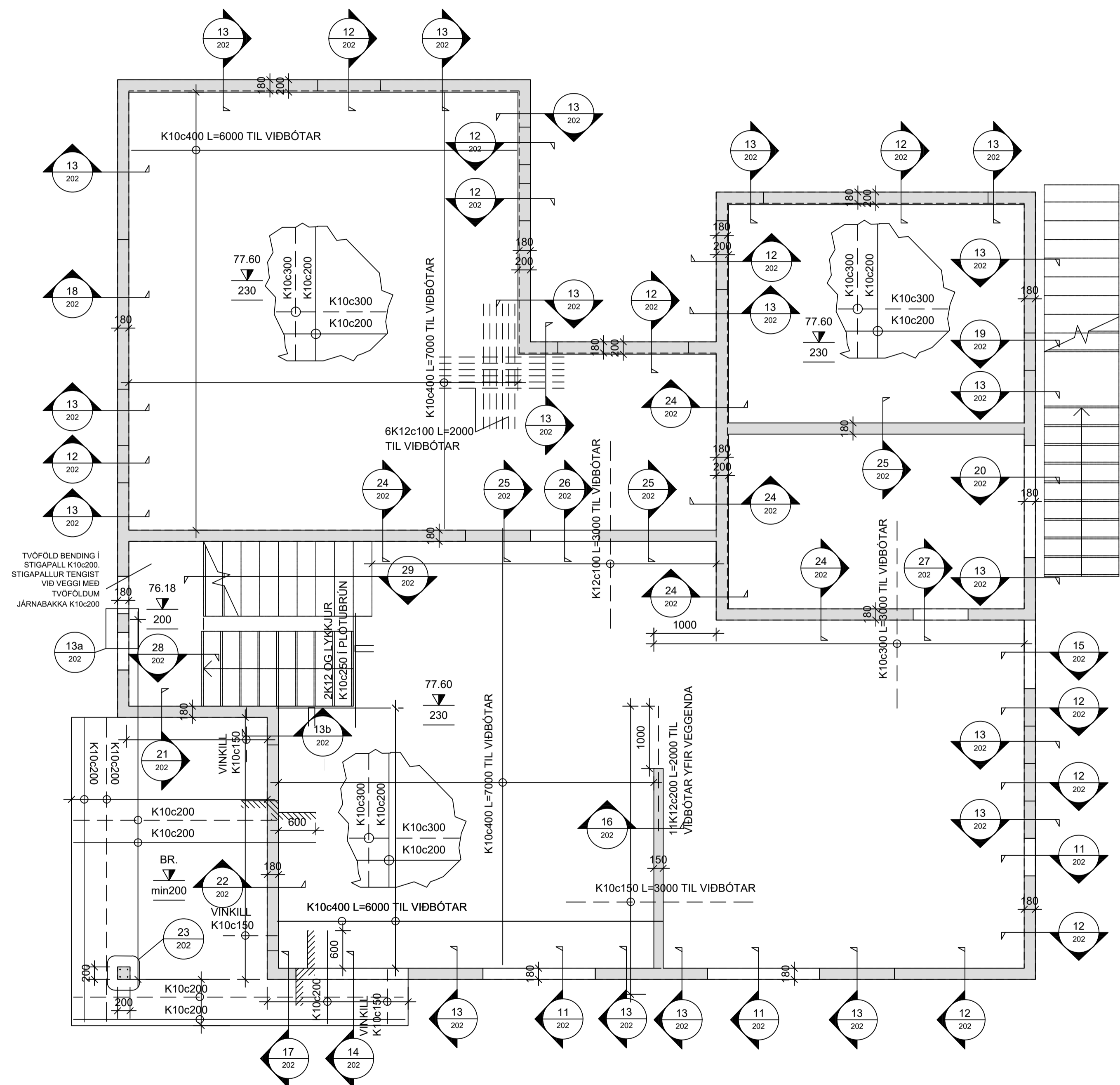
LOFTAPLATA 1 HÆÐAR, GRUNNMYND MKV. 3
