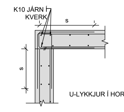
K3 LÁRÉTT KENNISNIÐ - VEGGHORN Mkv. 2
