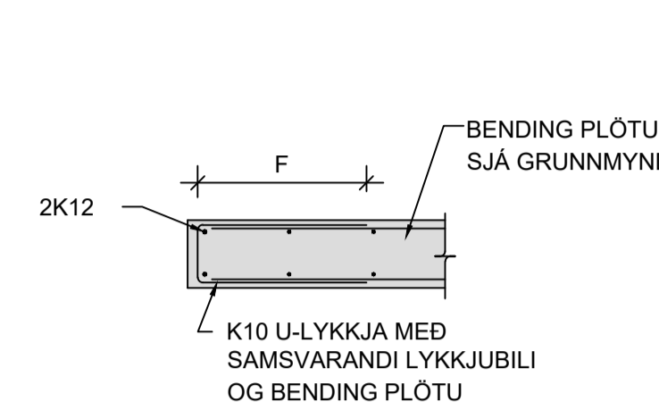
K2 LÓÐRÉTT KENNISNIÐ - PLÖTUBRÚN Mkv. 2
